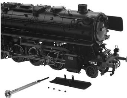
Abbildung 4: Windleitbleche & Befestigungsschrauben
